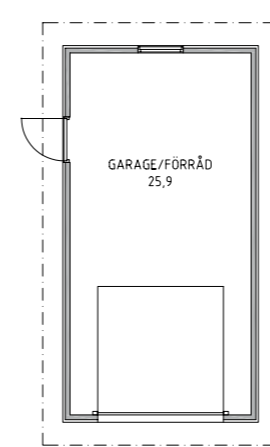
GARAGE MED FÖRRÅD GF 4-7 Byggarea: 29,1 m 2 B: 3,89 m L: 7,49 m
