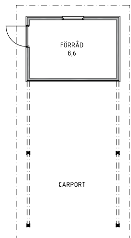
CARPORT MED FÖRRÅD CF 4-8 Byggarea: 33,6 m 2 B: 3,89 m L: 8,64 m
