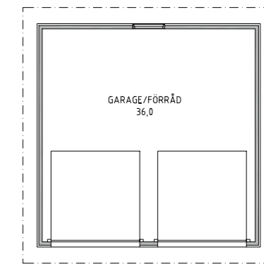
DUBBELGARAGE GG 6-6 Byggarea: 39,6 m 2 B: 6,29 m L: 6,29 m
