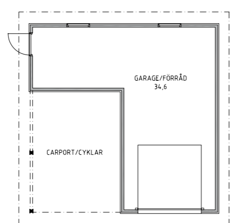
GARAGE, CARPORT OCH FÖRRÅD GCF 7-7 Byggarea: 56,0 m 2 B: 7,49 m L: 7,49 m
