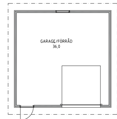
GARAGE MED FÖRRÅD GF 6-6 Byggarea: 39,6 m 2 B: 6,29 m L: 6,29 m
