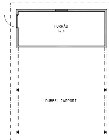
DUBBELCARPORT MED FÖRRÅD CCF 6-8 Byggarea: 54,3 m 2 B: 6,29 m L: 8,64 m
